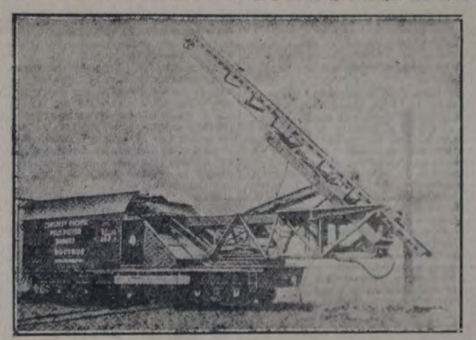
LA MAQUINA ATRAVESANDO LA VIA
