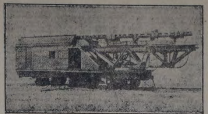
LA LOCOMOTORA DE HUNDIR POSTES. EN POSICION DE MARCHA
